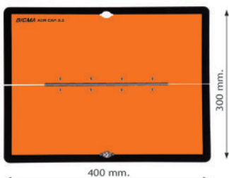
A.D.R. панель из нерж. стали, сгибаемая по горизонтали с петлей из нержавеющей стали, алюминий. Al: Алюминий
